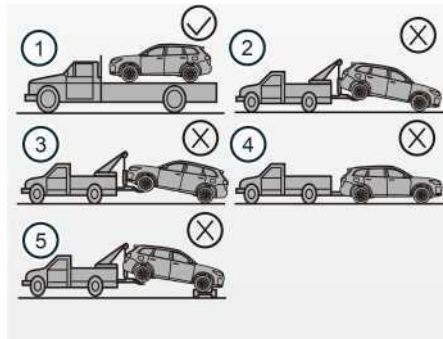
Иллюстрация: Погрузка автомобиля с помощью эвакуатора
