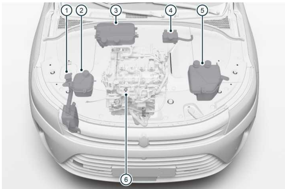
Иллюстрация: пространство капота автомобиля
