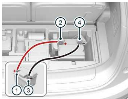
Иллюстрация: подсоединение проводов к аккумулятору
